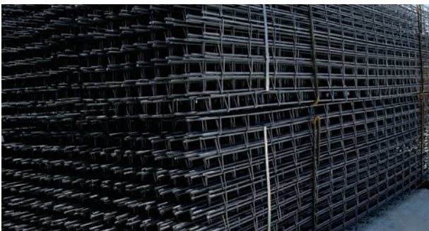
Trafer lattice girders / Reti Trafer Trafer-Gitter
