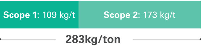
EMISSIONI SPECIFICHE DI CO 2eq /t (SCOPE 1 E 2) DELLE LAVORAZIONI A CALDO
