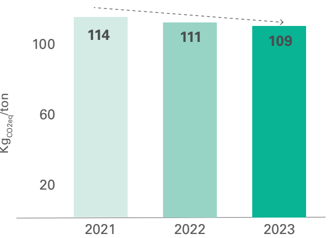
INTENSITÀ DELLE EMISSIONI DI CO 2eq (SCOPE 1) DELLE LAVORAZIONI A CALDO
