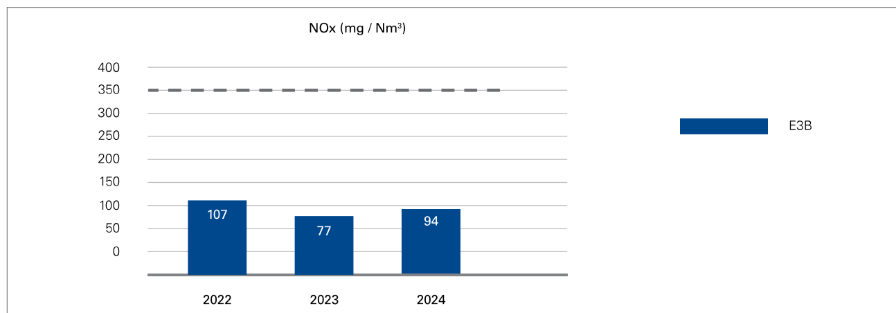
Figura 11.1 - Analisi relative NOx del camino E3B e concentrazione limite autorizzata (2022-2024)
