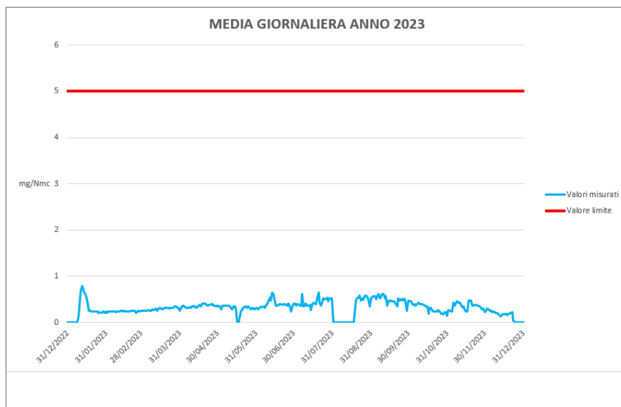
Figura 10.1 - Emissioni rilevate dallo SME nell'anno 2023
