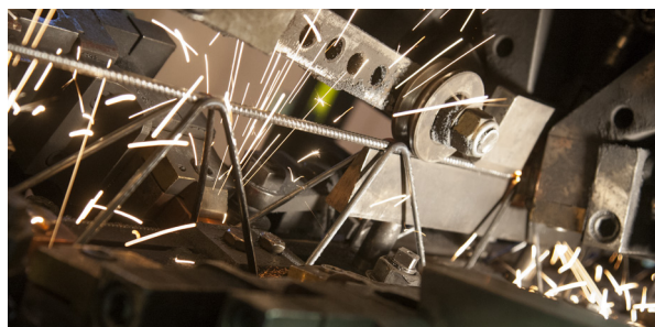
Figura 3.5 - Impianto Lavorazioni a Freddo (sezione tralicci)
