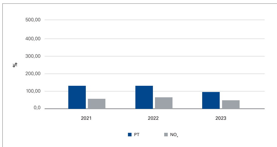
Figura 10.2 – Flussi di massa dei principali inquinanti emessi in atmosfera nel triennio 2021-2023, indicizzati rispetto al 2017.
