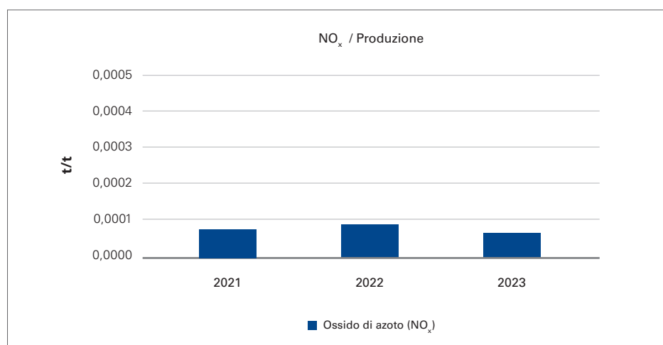
Figura 10.4 - Flusso di massa stimato di \text{NO}_x emessa su tonnellata di produzione nel triennio 2021-2023
