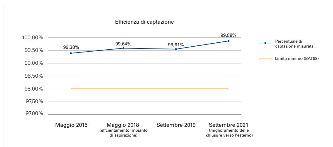
Figura 10.5 - Efficienza di captazione misurata e confronto con il limite minimo
