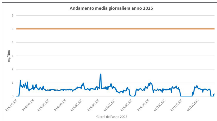
Figura 10.1 - Emissioni rilevate dallo SME nell'anno 2025
