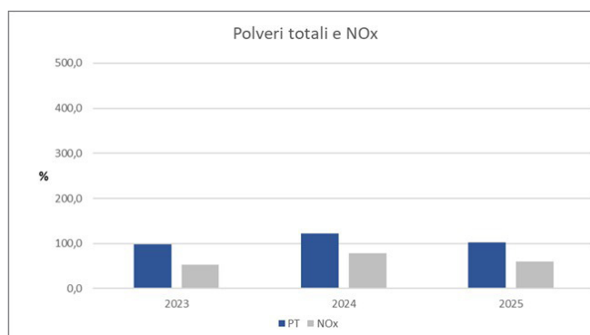
Figura 10.2 – Flussi di massa dei principali inquinanti emessi in atmosfera nel triennio 2023-2025, indicizzati rispetto al 2017.
