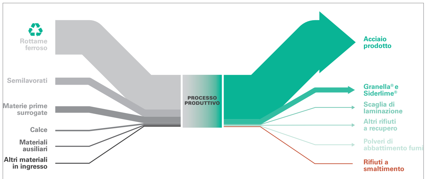
Figura 10.8 – Diagramma qualitativo dei flussi di materiale
